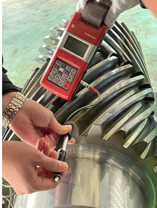
Corona y piñón de 13.5' x 20 para molino de bolas vendido a mina Mount Polley, imperial metals, Canada
